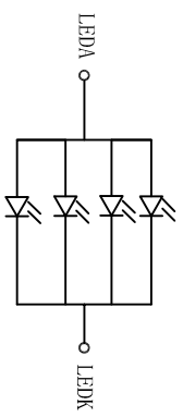
电路图 V=3.2V, I=20*4=80mA
